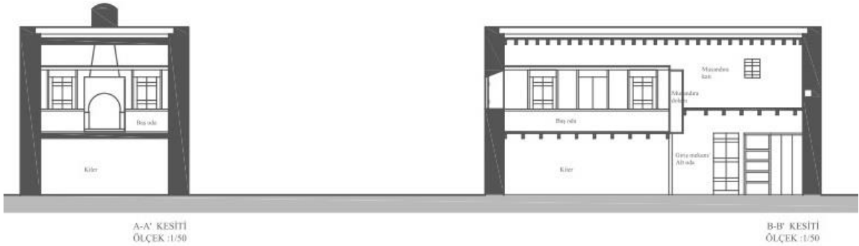
Şekil 6. Yalıkavak Dağbelen No:21, kesit görünümleri
