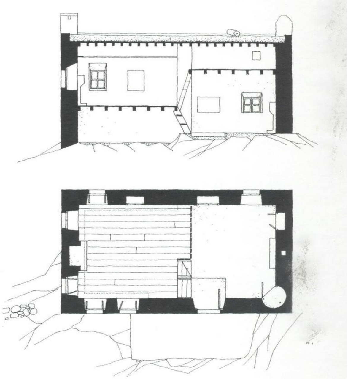
Şekil 1. Musandıralı eve ait kesit ve zemin kat planı [3]
