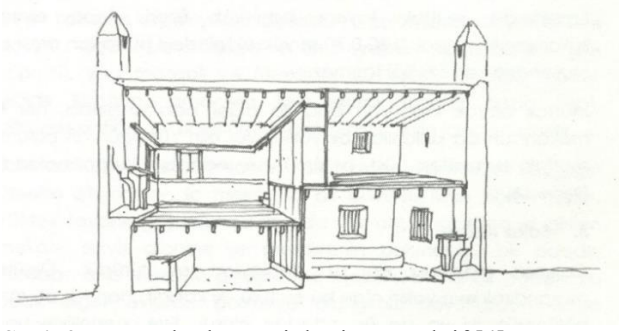
Şekil 2. Musandıralı eve ait kesit perspektif [4]
