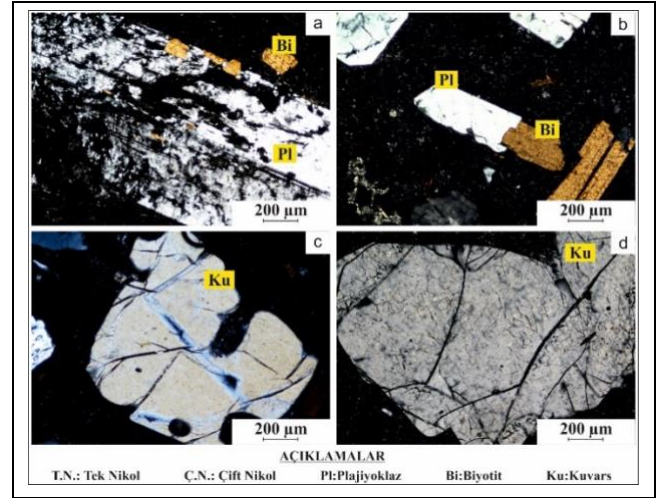
Şekil 3. İncelenen volkanitlerde gözlenen minerallerinin polarizan mikroskop altındaki görünümüleri.
