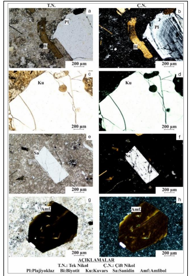
Şekil 4. İncelenen volkanitlerde gözlenen minerallerinin polarizan mikroskop altındaki görünümüleri.
