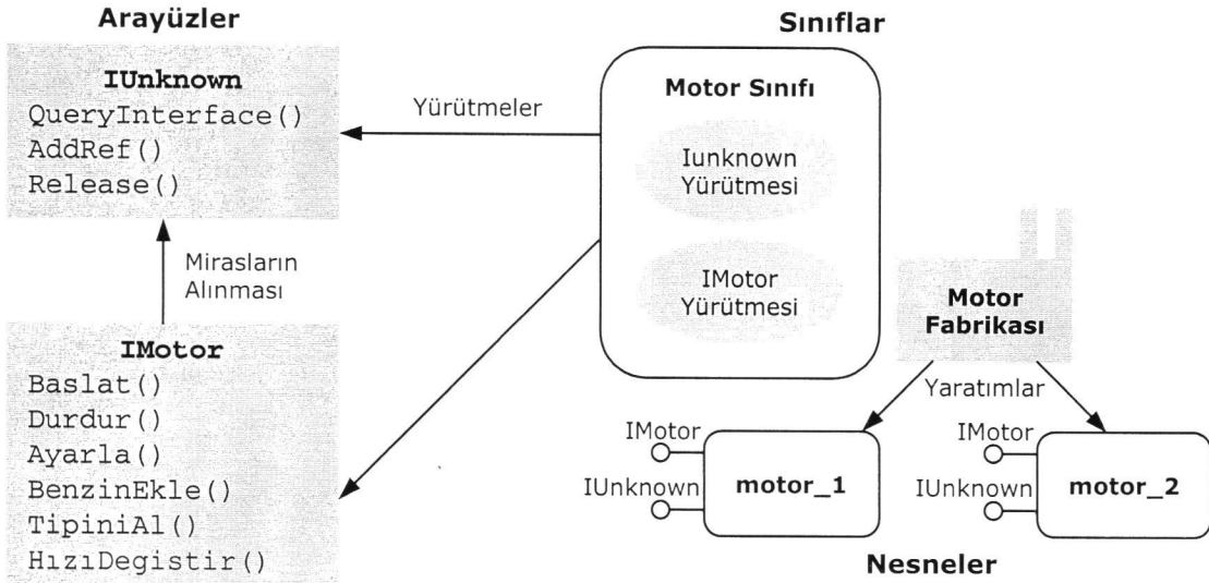
Şekil 7. Arayüzler, Sınıflar ve Nesneler
