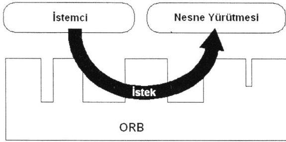
Şekil 2. ORB Üzerinden Gönderilen Bir İstek
