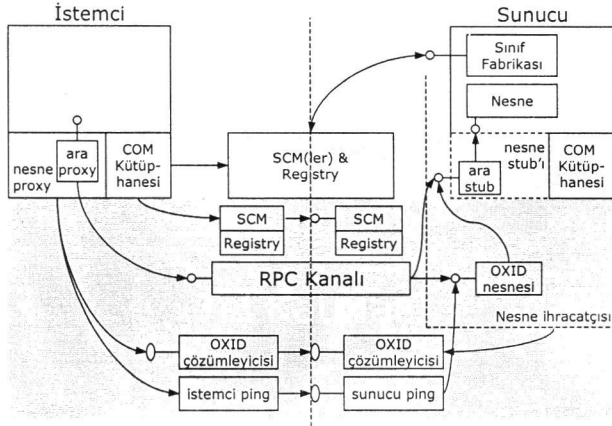
Şekil 10. DCOM Mimarisi
