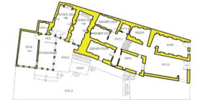
ZEMİN KAT PLANI
