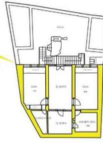
BİRİNCİ KAT PLANI
