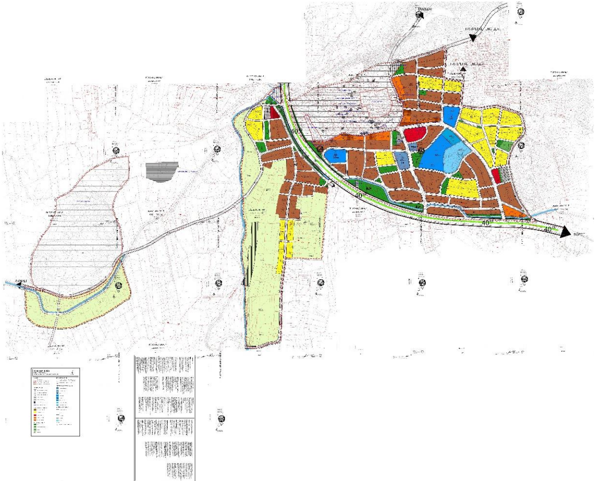
Şekil 7. Konuralp Koruma Amaçlı Revize İmar Planı (AKS Planlama ve Mühendislik Ltd. Şti. )
