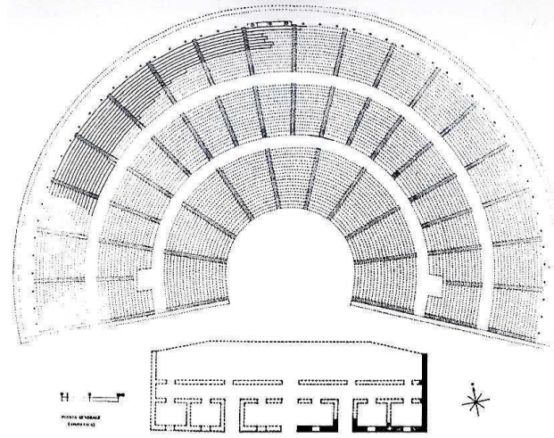
Şekil 5. Konuralp Tiyatro (1970 yılında B. Fernando tarafından yapılmış olan restitüsyon) (Zeyrek ve Çelik 2005: 41-42)
