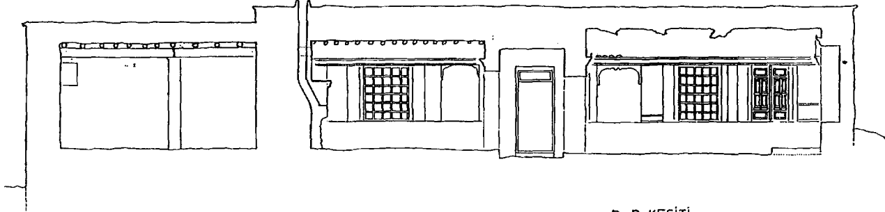
B. B KESİTİ
