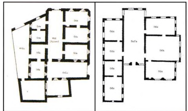
Çizim : 1 Resul Özkul Evi zemin kat plânı
