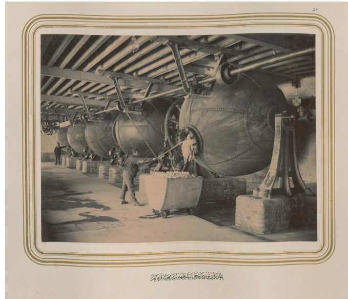
Fotoğraf 4: Kâğıt Hamurunu 100 Derecelik Sıcaklıkla Temizleyen Dönen Kazanlar
