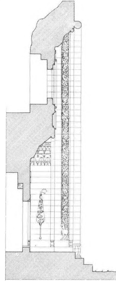
A-A Kesiti
