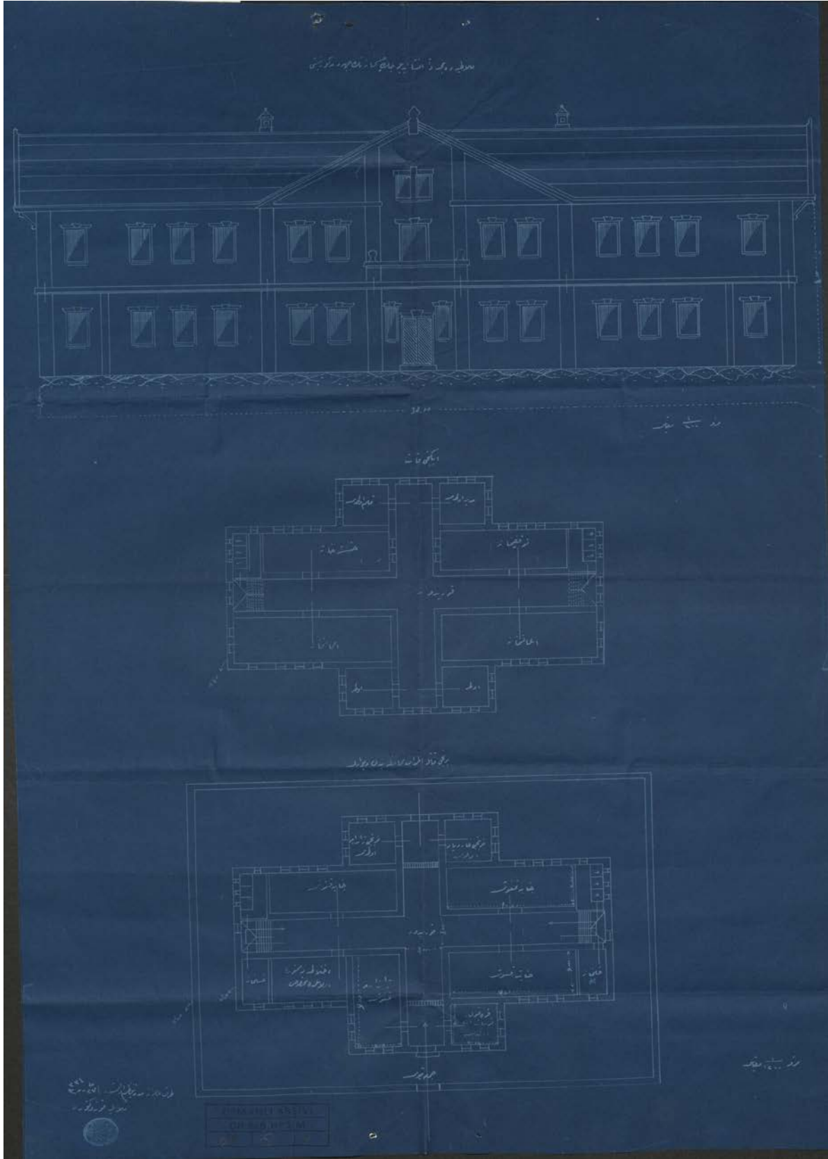
Ek-3: Eskisi yıkılmaya yüz tuttuğu için yenisinin yapılması gerektiği ifadesiyle çizilen yeni Malatya merkez hapishanesi projesi. BOA. DH. MB. HPS. M. 55/8, 25 L 1336 (3 Ağustos 1918).
