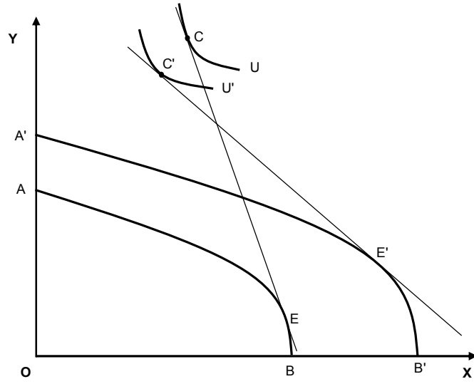
Şekil 1: Yoksullaştırıcı Büyüme
