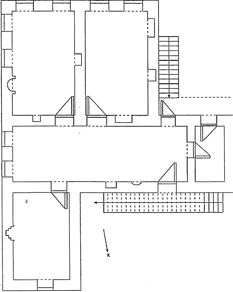
Abid Ağa Konağı 1. Kat (Selamiye) Planı.
