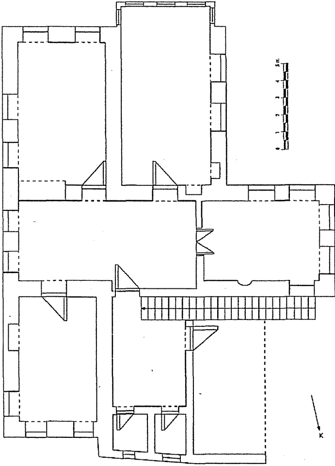
Abid Ağa Konağı, 2. Kat (Haremlik) Planı.
