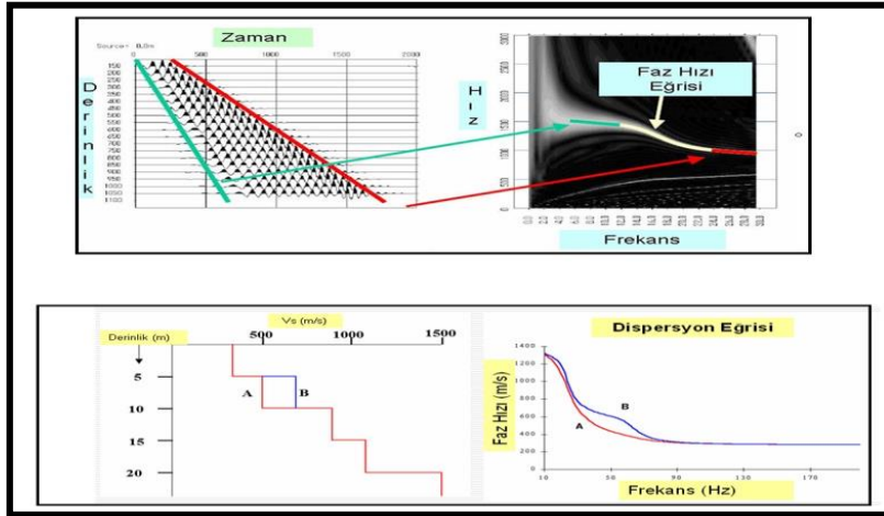
Şekil 6. Yüzey dalgalarının dalga formu ve dispersiyon eğrisi ve ters çözümü ile elde edilmiş Vs hız profili
