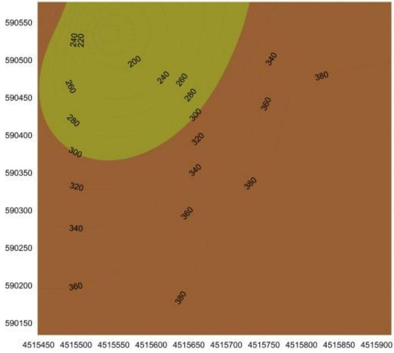
Şekil 7. Kesme dalgası hızlarının ( V_s ) dağılımı
