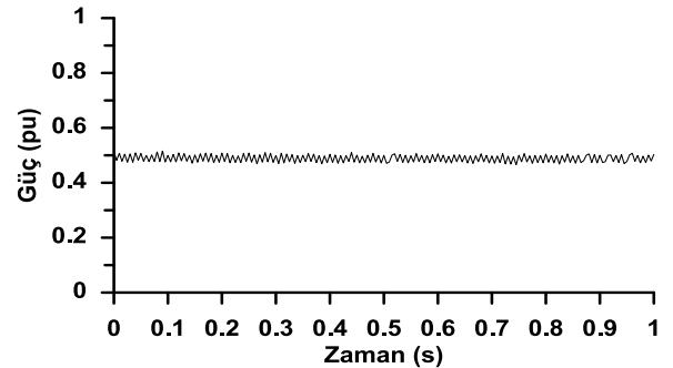
Şekil 3. Yarı yükte arızasız çalışma durumunda asenkron generatörün ani gücü (Instantaneous power of the half loaded asynchronous generator in unfaulty condition)
