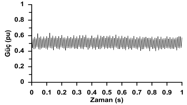
Şekil 7. Yarı yükte orta derecede mekanik dengesizlik durumunda asenkron generatörün ani gücü (Instantaneous power of the half loaded asynchronous generator in middle mechanical unbalanced condition)
