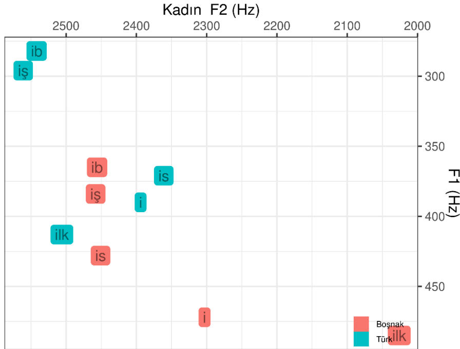
Şekil 6: /i/ ünlüsüne ait kadın formant grafiği. Kırmızılar Boşnak 25 kadın öğrenciye ait ortalama değer, maviler ise Türkçe ana dil konuşuru 3 kadına ait ortalama değeri göstermektedir.
