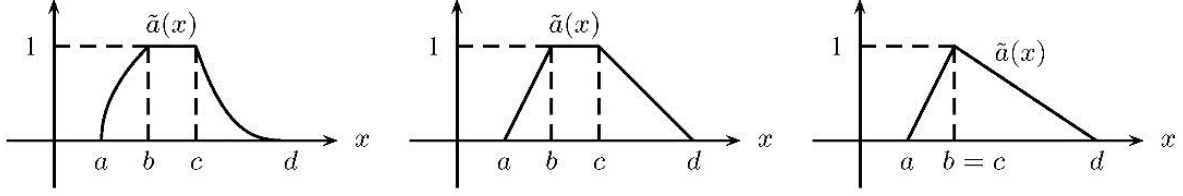
Şekil 3: Sırasıyla LR, yamuk ve üçgensel fuzzy sayılar
