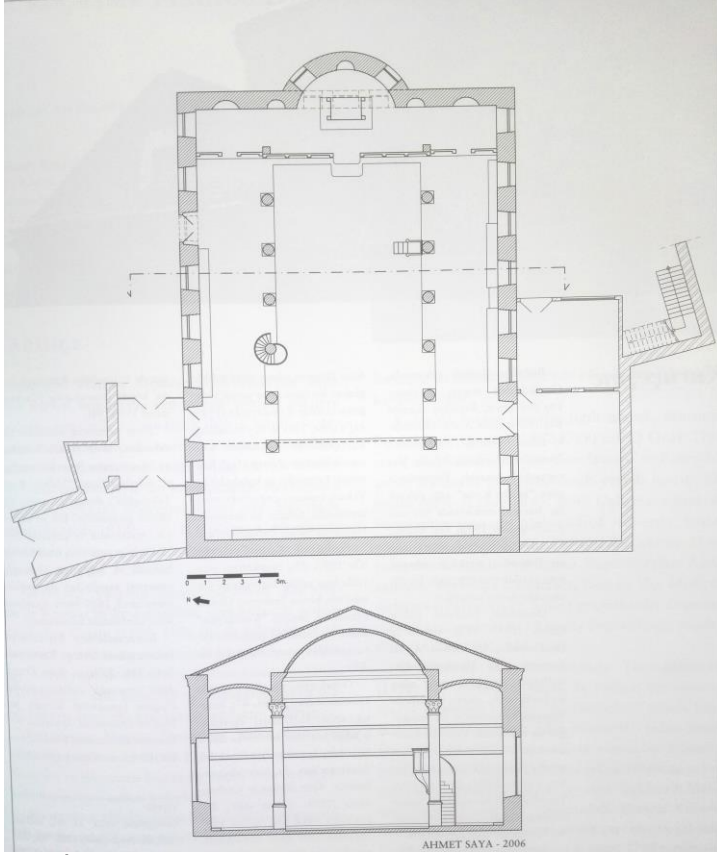
Resim 8. İstanbul Hagios Phokas Kilisesi, Plan ve Kesit (Karaca, 2008: 389)
