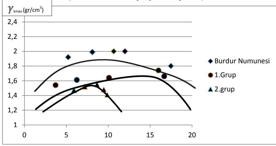
Şekil 1. Standart Kompaksiyon Denei Sonuçları
