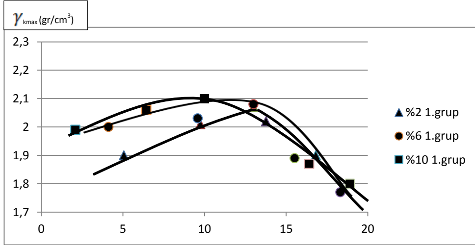
Şekil 2. Birinci Grup Mermer Kırığı Katkılı Standart Kompaksiyon Denei Sonuçları
