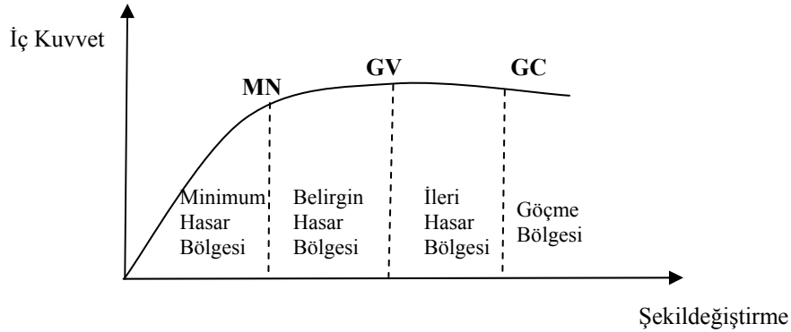
Şekil 1. Hasar sınırlarının ve bölgelerinin grafiksel gösterimi.
