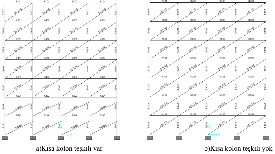
Şekil 2. Seçilen örnek düzlem çerçeve binaların şematik gösterimi.
