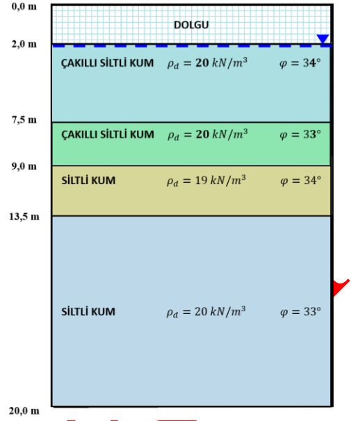
Şekil 3. Adapazarı kesiti (Adapazarı cross section)
