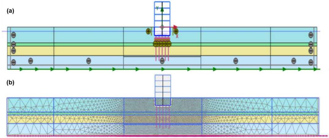
Şekil 5. (a) Sonlu eleman modeli (Finite element model), (b) Oluşturulan ağ, (Generated mesh)
