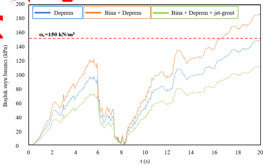
Şekil 10. S3 noktasında oluşan boşluk suyu basınçlarındaki değişim (Change in pore water pressures at the S3)
