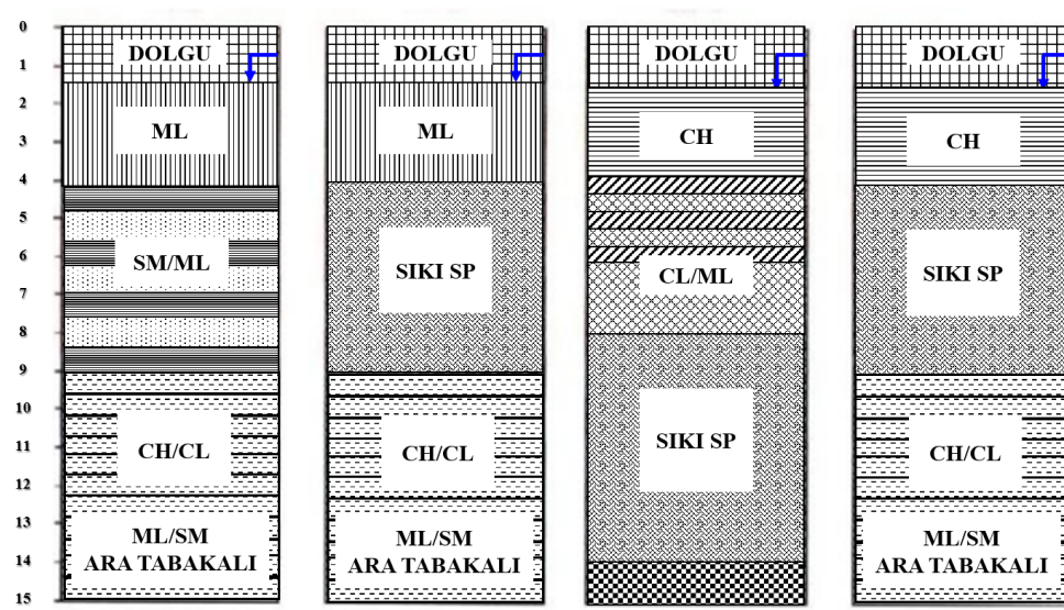
Şekil 1. Adapazarı Kent Merkezi zemin profilleri (Adapazarı City Center soil profiles) [28]
