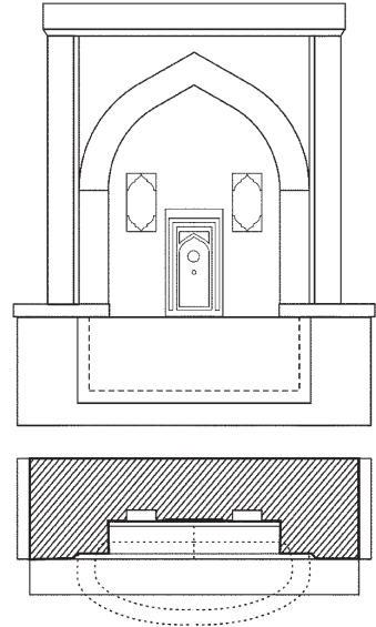
29. Kemer Aynalı Çeşme Plan ve Cephe Çizimi
