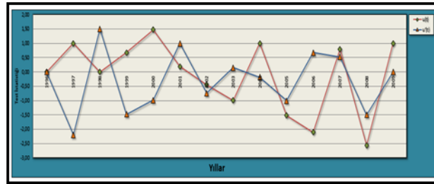
Şekil 2. Trend olmaması durumunda u(t) - u'(t) grafiği.
