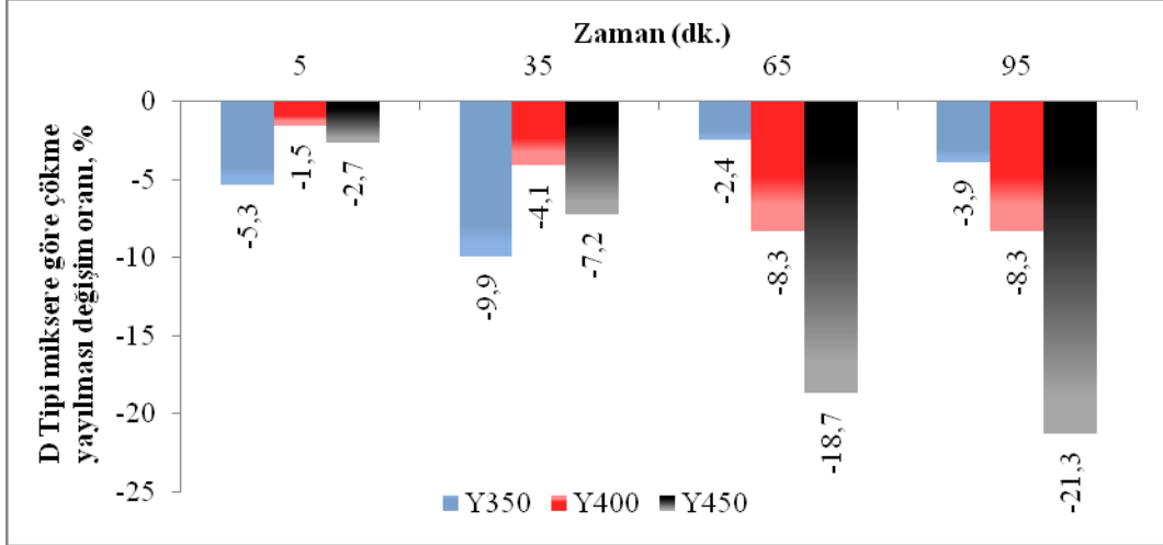
Şekil 6. D tipi mikserde Y tipi mikserin çökme yayılması değişim oranları
