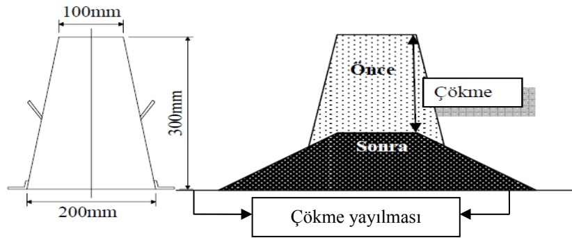
Şekil 3. Çökme ve çökme yayılmasının şematik olarak gösterimi (Özel, 2007)
