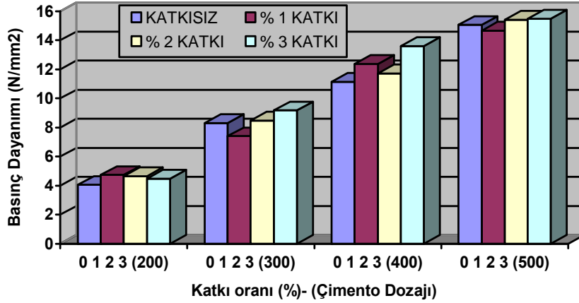
Şekil 4. 7. günde katkı kullanım oranına bağlı basınç dayanımı değişimi
