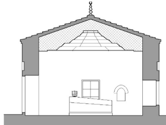
Çizim-1. Memi Baba Türbesi'nin rölöve ve restitüsyon önerileri ● özgün duvarlar ● ilaveler (Mehmet Emin Yılmaz - 02.06.2018)
