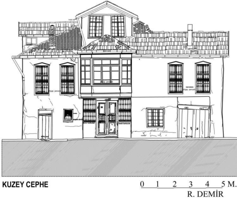
Çizim 2: Abdülkadir Dolmacı Evi Görünüşü (R. DEMİR)
