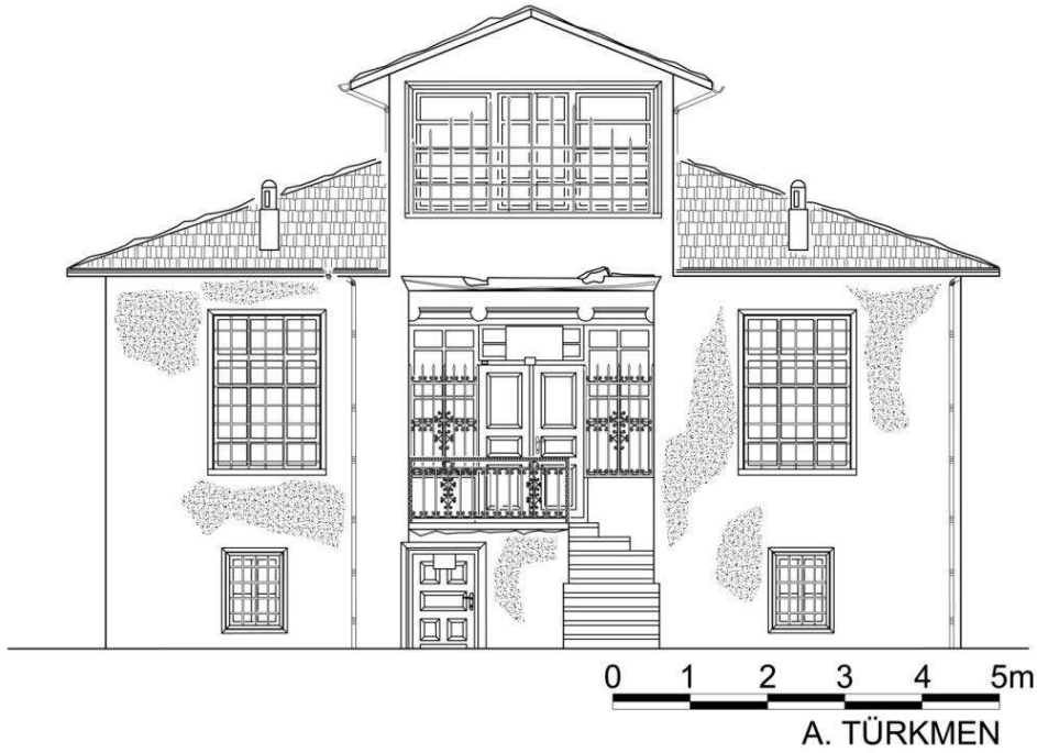
Çizim 3: Selçuklu Araştırmaları Merkezi Evi Görünüşü (A. TÜRKMEN)
