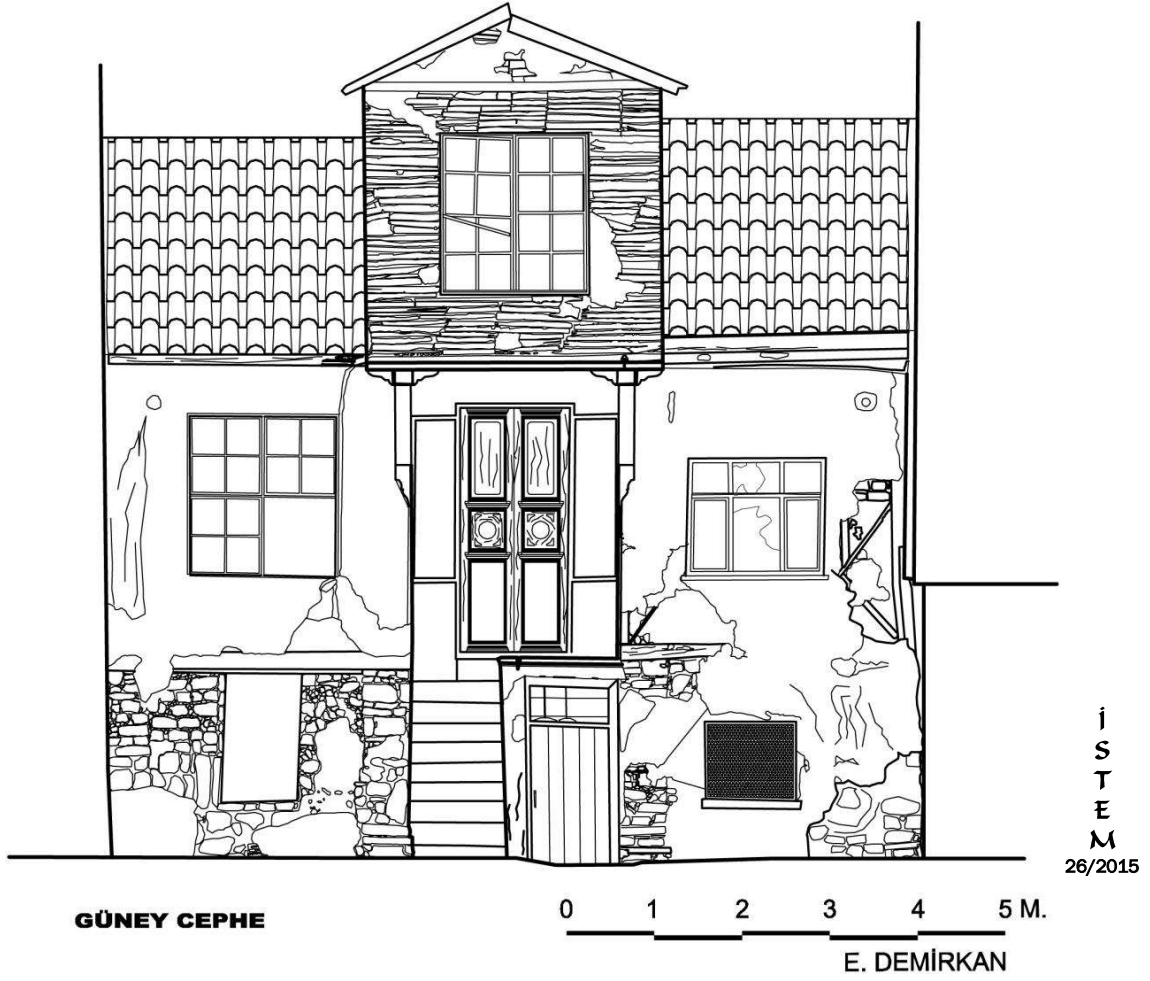
Çizim 5: Perihan Özkarakoç Evi Görünüş (E. DEMİRKAN)
