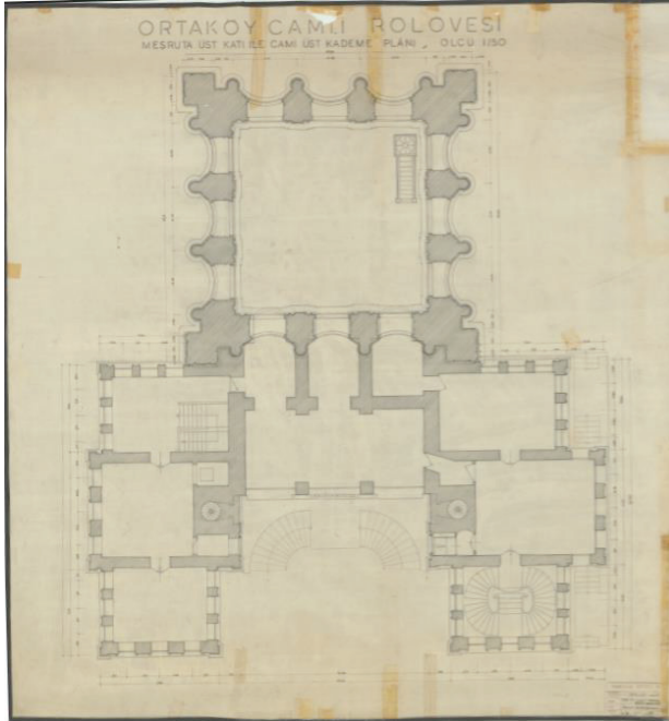
Çiz.2: Ortaköy Camii İkinci Kat Planı (Vakıflar Genel Müdürlüğü)
