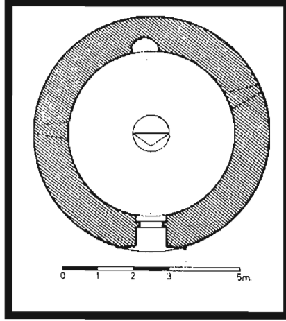
Çizim 3 : Söylemez Ana Kümbeti Planı (R. H. Ünal'dan)
