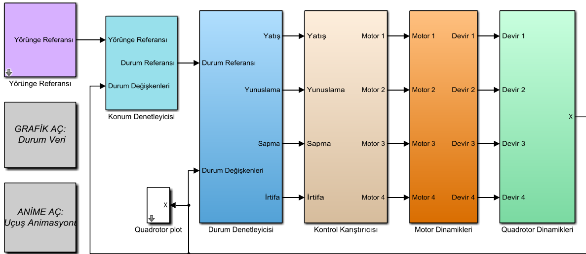
Şekil 10. Doğrusal olmayan model için simülük blok diyagramı (Block diagram for nonlinear simulink model)
