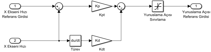
Şekil 7. X eksen PD denetleyicisi (PD controller for X axis)
