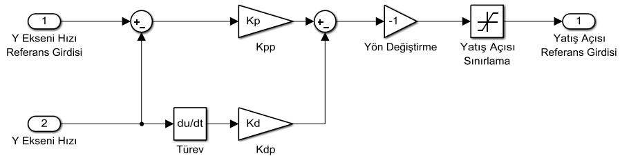
Şekil 8. Y eksen PD denetleyicisi (PD controller for Y axis)
