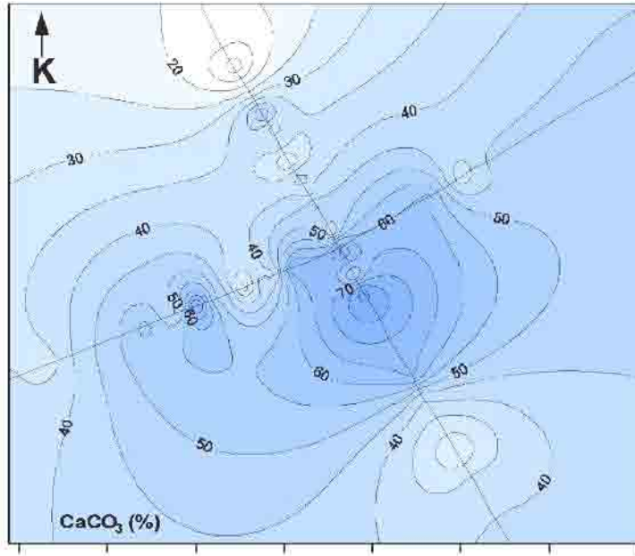
Şekil 15. Çalışma alanı yüzey çökeltilerinde CaCO 3 miktar dağılımı.
