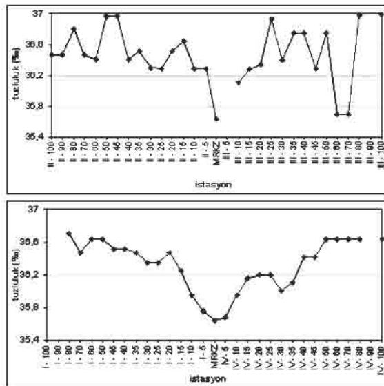
Şekil 11. Örnekleme hatları boyunca dip suyunda tuzluluk değişimi.
