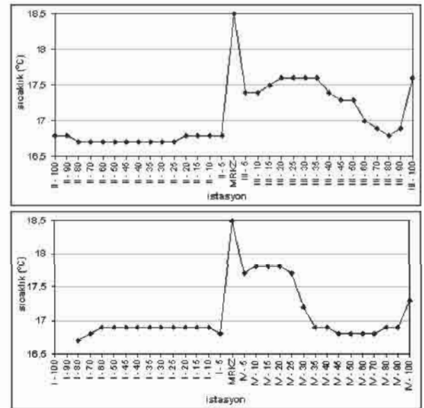
Şekil 9. Örneklem hatları boyunca dip suyu sıcaklığı değişimi.
