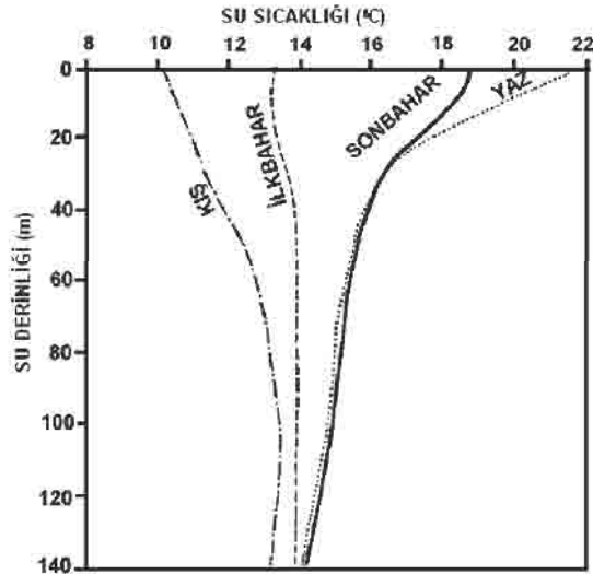
Şekil 4. Saros Körfezi mevsimlik su sıcaklığı (Eryılmaz ve Yücesoy Eryılmaz, 2003).
