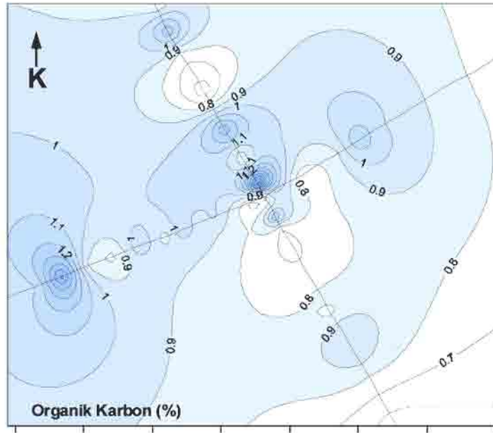
Şekil 16. Çalışma alanı yüzey çökeltilerinde organik karbon miktar dağılımı.
