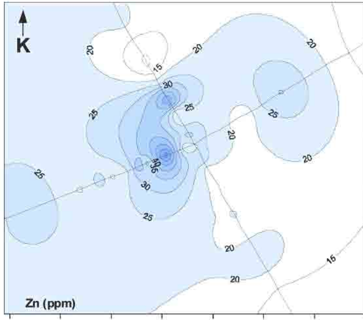
Şekil 19. Çalışma alanı yüzey çökellerinde Zn dağılımı.
