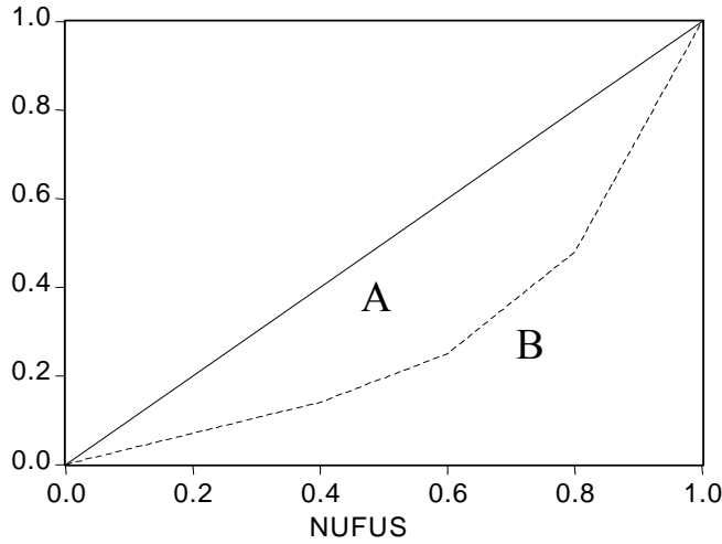
Şekil 1. Lorenz Eğrisi
