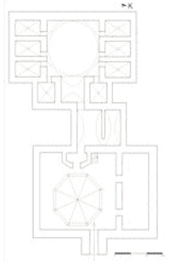
Plan 7: Erzurum (Pastırmacı-Fuadiye) Hamamı
