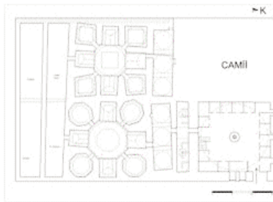
Plan 5: Boyahane Hamamı
