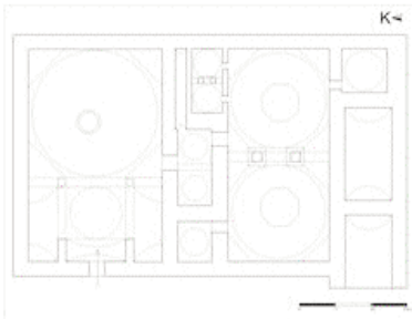
Plan 9: Çifte Göbek Hamamı
