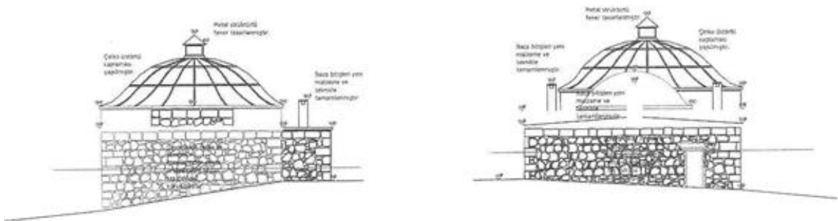
Çizim 2: Gümrük Hamamı (V.G.M'den)
