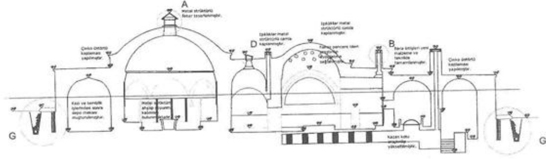
Çizim 3: Gümrük Hamamı Kesiti (V.G.M'den)
