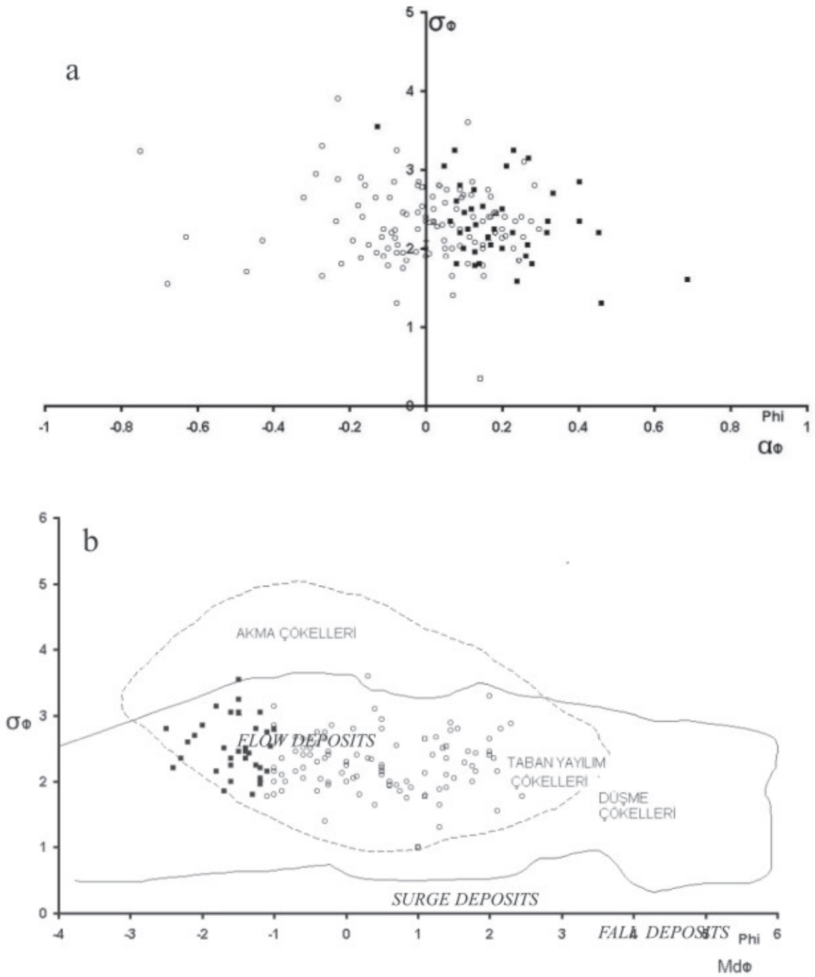
Şekil 11. a) \sigma_\phi karşı \alpha_\phi dağılım diyagramı. b) \sigma_\phi 'ye karşı Md_\phi dağılım diyagramı (Walker, 1971). ■: lapilli ve blok ağırlıklı taban yayılım fasiyesi ve o: kül ağırlıklı taban yayılım fasiyesi
