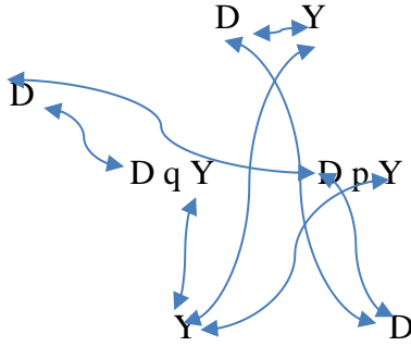
Şekil 2. \sim (p \sim q) tuncesi
