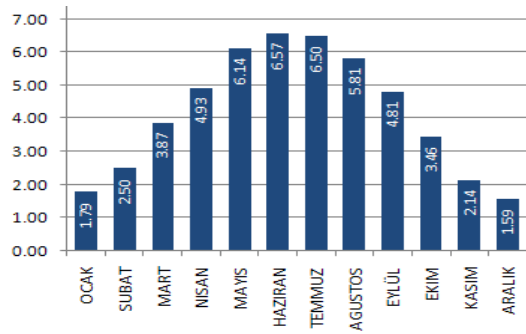
Şekil 2a. Türkiye global radyasyon değerleri (kWh/m 2 -gün)
