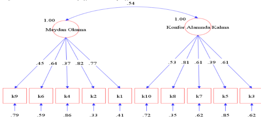
Konfor Alanı Yönelim Ölçeği DFA Diyagramı
