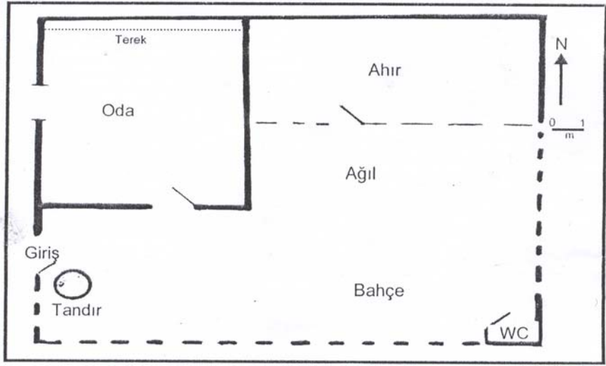
Şekil 6. Binbaşeminbey Yaylasındaki Bir Yayla Konutuna Ait Plan.
