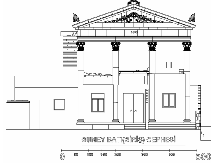
Çizim 3: Ayazma Kilisesinin giriş cephesi
