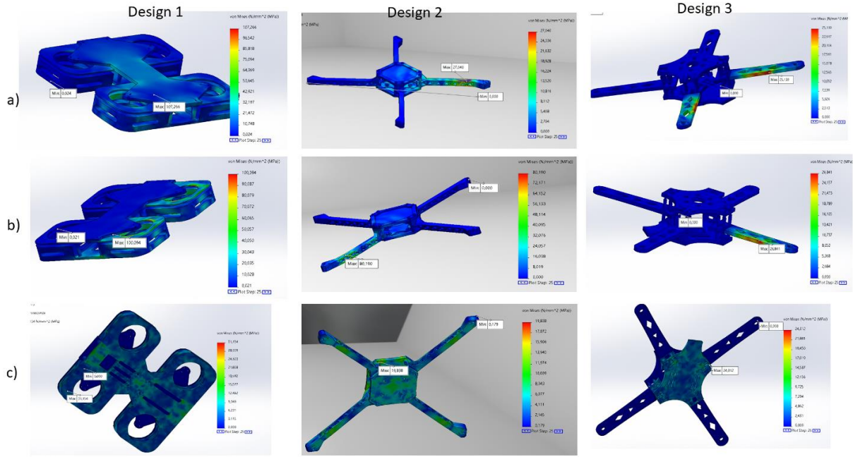
Figure 3. Von Mises stress analysis of Drone Frame Designs a) Direction 1, b) Direction 2, c) Direction 3 (Drone Gövde Tasarımlarının Von Mises Gerilme Analizi a) Yön 1, b) Yön 2, c) Yön 3)
