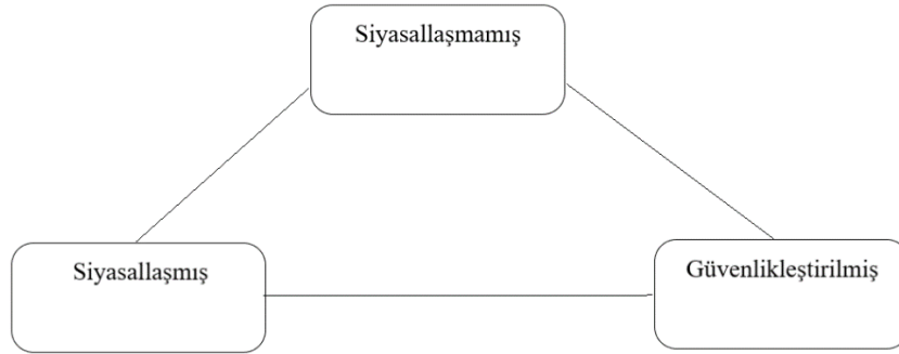
Şekil 1: Güvenikleştirme Döngüsü
