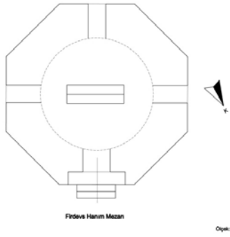
Çizim 4: Firdevs Hatun Türbesi Planı
