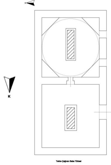
Çizim 2: Çayırın Baba Türbesi Planı
