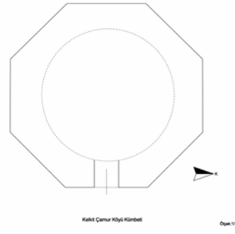
Çizim 5: Çamur Köyü Kümbeti Planı
