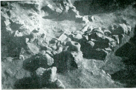
Res. 10 — Kalkolitik II. tabaka mimarisinden parçalar ve yerinde kalan Kapısögesi mili. Fig. 10 — Buildings of second chalcolithic level (Door-socket in situ).
