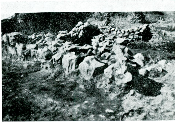
Res. 4 — Kazı alanı güneyinde Frig çağı duvarları Fig. 4 — Phrygian walls, southern part of excavated area
