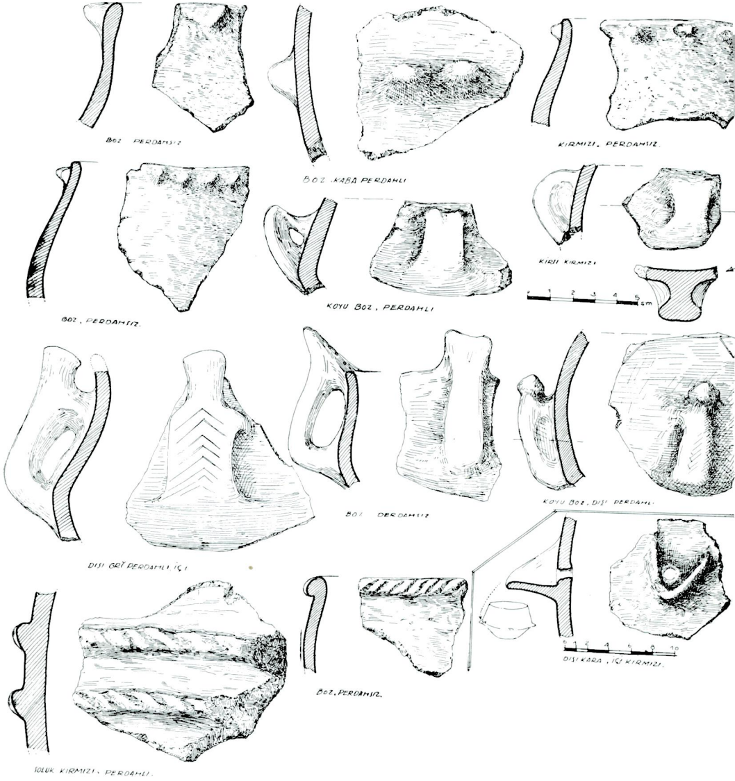
Res. 47 — Büyük Güllücek. Kulp çeşitleri; Göğde, kenar süsleri ve akıtacak. Fig. 47 — Types of handles; decoration of bodies and rims; spouts:
