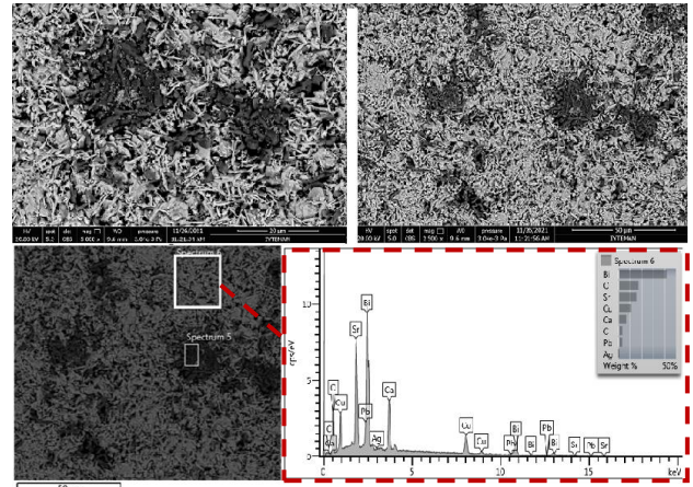
Şekil 3. B ( x=0.05 ) örneğinin farklı büyütme görüntüleri. Altta satır ise B-örneğinin EDX analiz sonucu.
