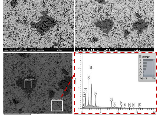
Şekil 2. Soldan sağa doğru A-örneğinin 5000x ve 2500x büyütme görüntüleri. Altta satır ise A-örneğinin EDX analiz sonucu.
