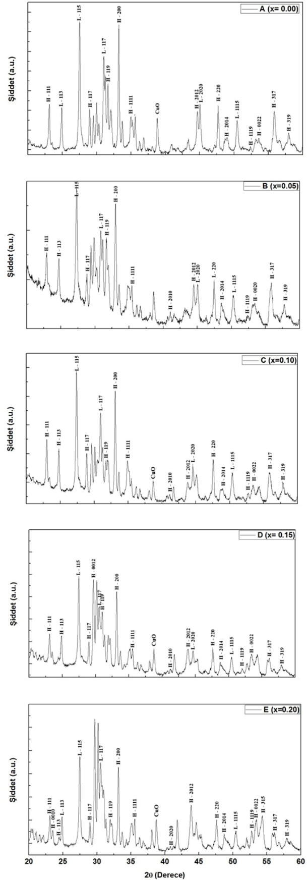
Şekil 1. Bi_{1.7}Pb_{0.3-x}Sb_xSr_2Ca_2Cu_{3-x}Ag_xO_y ( x=0.00-0.20 ) örneklerinin XRD grafikleri.
