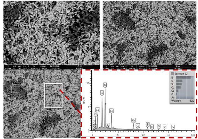
Şekil 4. C ( x=0.10 ) örneğinin farklı büyütme görüntüleri. Altta satır ise C-örneğinin EDX analiz sonucu.
