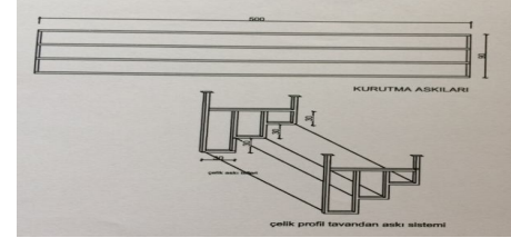
Şekil 14. Kurutma Alanı ve Askılık Planı.
