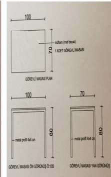
Şekil 9. Görevli Masası Planı
