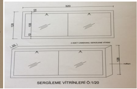
Şekil 12. Sergileme Vitrinleri Yan Kısım ve Orta Kısım Planı.
