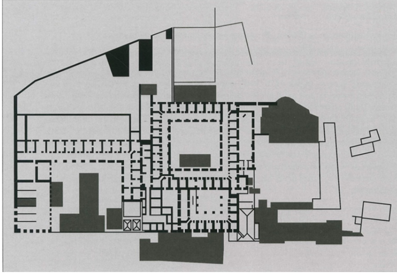
Fig. 8. İbrahim Paşa Sarayı'nın yeniden yapımından önce 1939'da Sedat Çetintaş tarafından çizilmiş planı (Atasoy 2012, 110)
