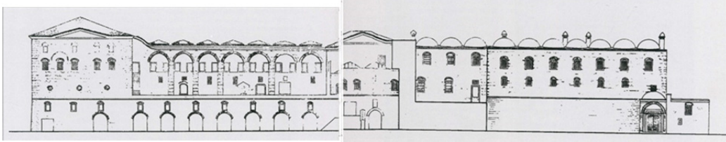
Fig. 4. İbrahim Paşa Sarayı'nın At Meydanı'na bakan cephesinin Y. Mimar Ertuğrul Eğilmez ve Y. Mimar Fatin Uluengin rölövesi (Atasoy 2012, 110)
