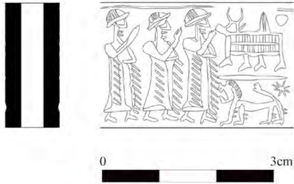
Figür 4. Elbistan Karahöyük silindir mührü ve baskısının çizimi
