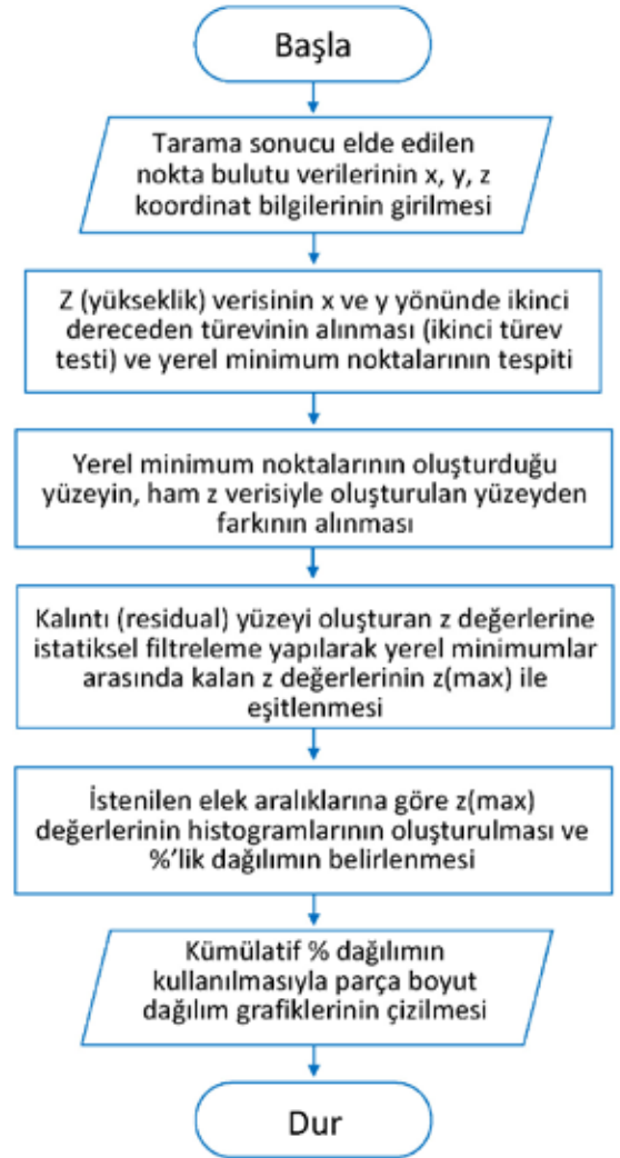
Şekil 6. MATLAB yazılımı ile tane boyu dağılımı belirlenmesinde uygulanan algoritma
