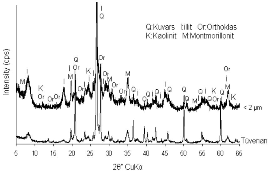
Şekil 2. İncehisar-Afyon kiline ait XRD grafiği.
