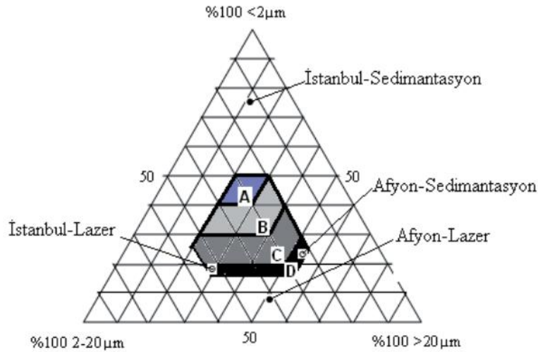
Şekil 9. Numunelerin boyut dağılımlarına göre Winckler's diyagramındaki konumları
