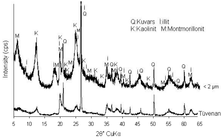
Şekil 3. Şile-İstanbul kiline ait XRD grafiği.
