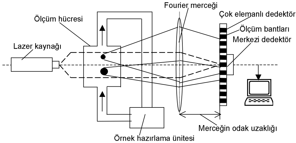
Şekil 1. Lazer kırınım cihazının genel şeması (Özer ve Orhan, 2007).
