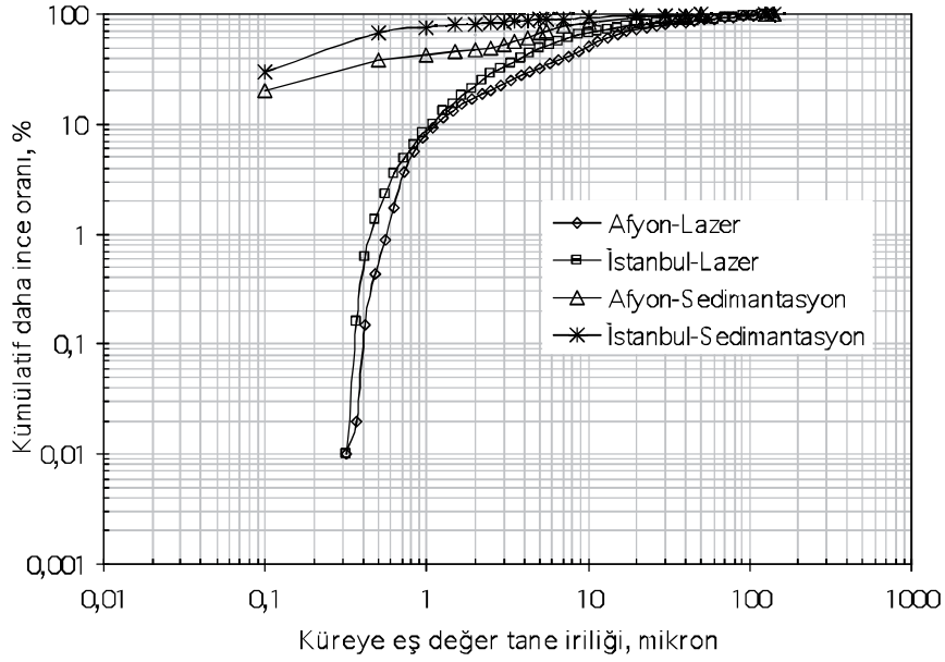
Şekil 10. Numunelerin 0-125µm fraksiyonunun iki yöntemle belirlenen küreye eş değer tane iriliği dağılımı.
