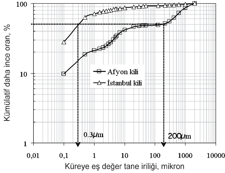
Şekil 8. Numunelerin X-ışınları sedimantasyon yöntemiyle belirlenen (<125µm fraksiyonu için) küreye eş değer tane iriliği dağılımı.
