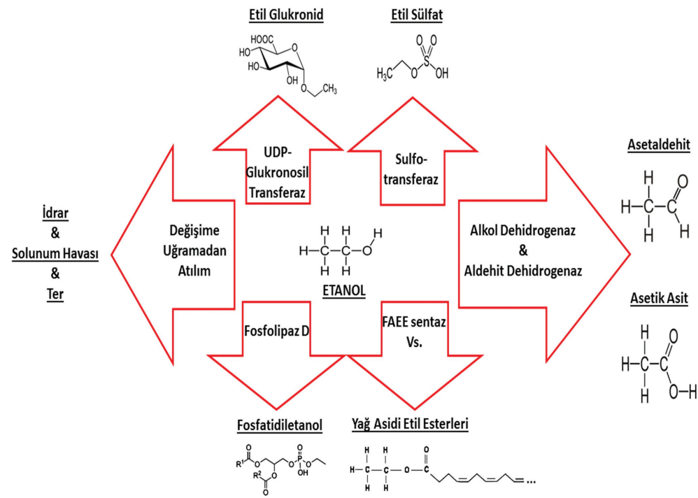
Şekil 1: Etıl alkolün metabolik yolları
